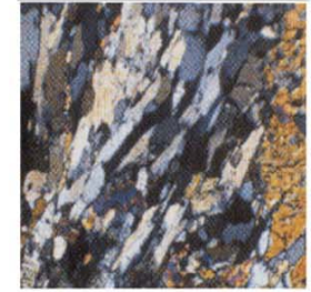
Glaucophane Amphibole bleue observée en lumière polarisée (polarisée + analysée)
