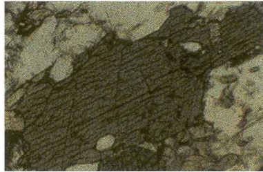
Hornblende Amphibole brune observée en lumière naturelle (polarisée)
