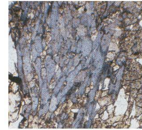
Glaucophane Amphibole bleue observée en lumière naturelle (polarisée)
