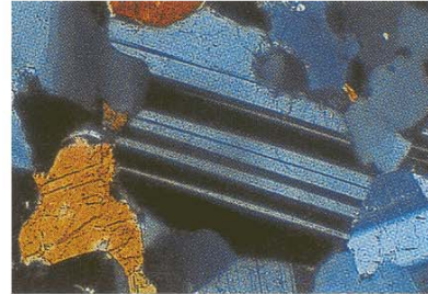
Feldspath plagioclase observé en lumière polarisée (polarisée + analysée)
