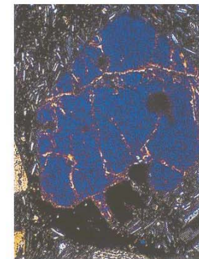
Péridot observé en lumière polarisée (polarisée + analysée)
